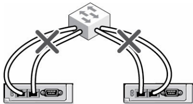
图 3: CMC 网络布线错误 - 2 个 CMC
